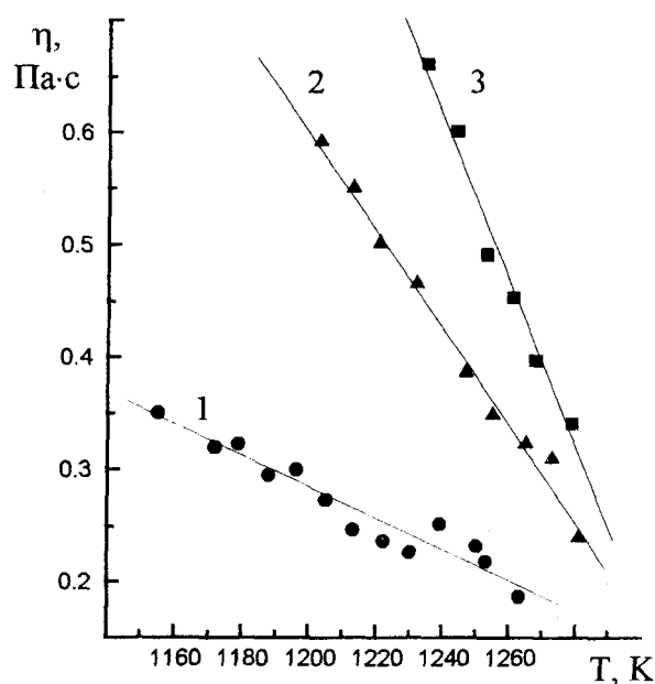
Рис. 2 - Зависимости вязкости расплавов на основе флюса \text{BaO-BaF}_2\text{-B}_2\text{O}_3\text{-PbO} от температуры
