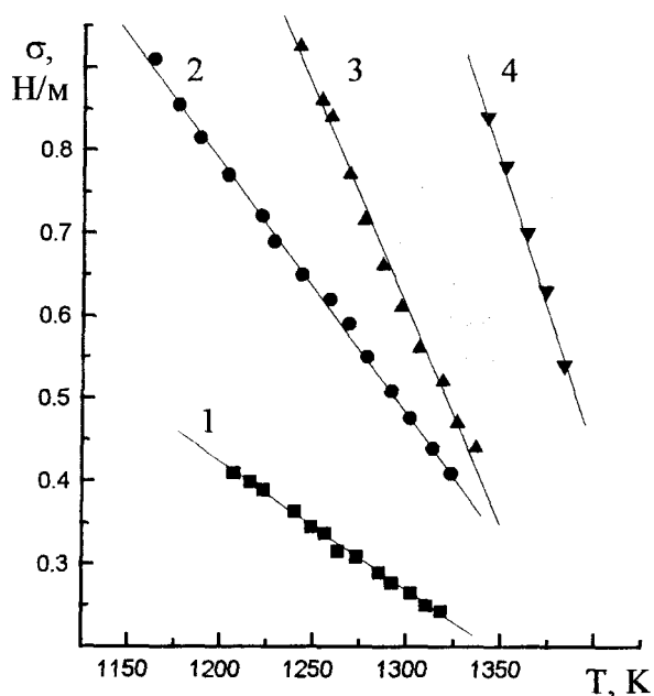
Рис. 1 - Зависимости поверхностного натяжения расплавов на основе флюса \text{BaO-BaF}_2\text{-B}_2\text{O}_3\text{-PbO} от температуры
