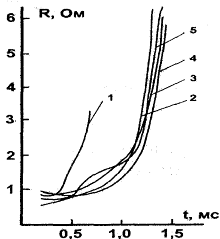
Рис. 4. Временные зависимости сопротивления канала разряда при U_0 = 5 кВ, L = 0,3 мГн, S = 145 мм и емкостях накопителя: 1 – 150 мкФ; 2 – 1,05 мФ; 3 – 1,50 мФ; 4 – 2,25 мФ; 5 – 3,0 мФ
