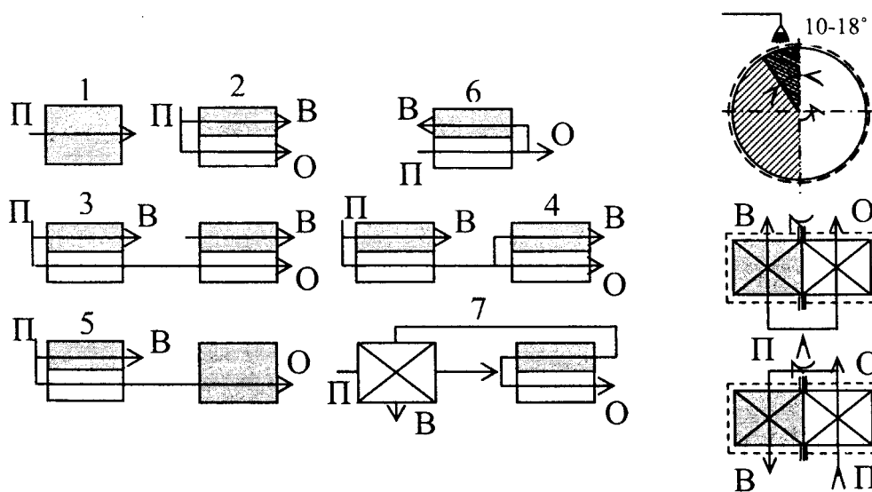
Рис. 1.Б. Непрямые испарительные охладители НИО совмещенного типа (1 – прямое испарительное охлаждение). Обозначения: 2 – одноступенчатые НИО; 6 – регенеративная схема; 3-5, 7 – двухступенчатые НИО; 8 – НИО с насадкой вращающегося типа
