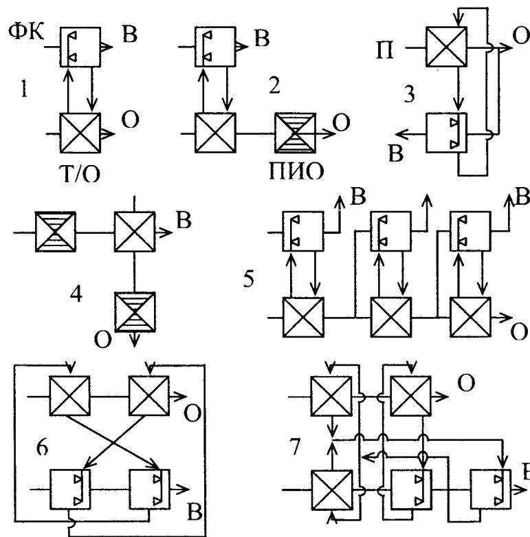
Рис. 1.А. Непрямые испарительные охладители НИО раздельного типа. Обозначения: 1 – 4 одноступенчатые НИО; 5 – 7 многоступенчатые НИО; 3, 6 и 7 – регенеративные охладители; П, О, В – полный, основной и вспомогательный воздушные потоки, соответственно; ФК – форсуночная камера; Т/О – теплообменник; ПИО – испарительный охладитель прямого типа
