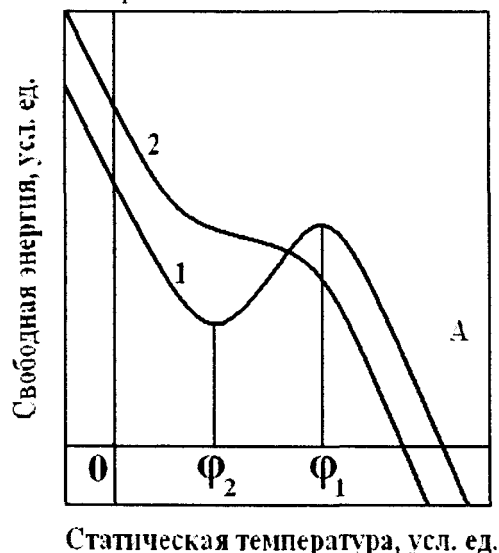
Рис. 1. Основные варианты графиков зависимости свободной энергии от статической температуры: \varphi_1 , \varphi_2 – значения статической температуры соответствующие максимуму и минимуму свободной энергии, А – область перехода к аморфному состоянию
