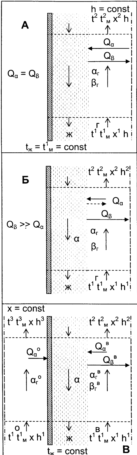
Рис. 3. К моделированию процессов совместного теплообмена при испарительном охлаждении
