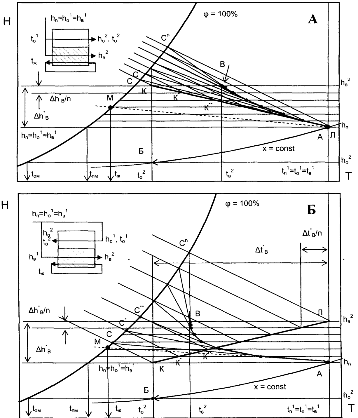
Рис.4. Изображение процесса в НИО на H-T диаграмме влажного воздуха. А – процессы в НИО при прямоточной схеме движения основного и вспомогательного воздушных потоков; Б – процессы в НИО при противоточной схеме движения воздушных потоков.
