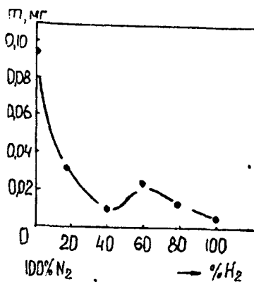
Рис. 2. Зависимость ионной эрозии титана от состава смеси азота с водородом (50 кэВ) при 850°С
