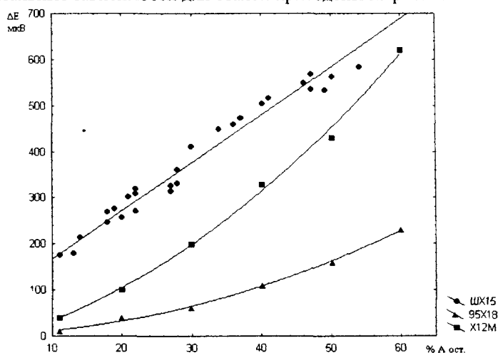
Рис.4. Зависимость фазочувствительной составляющей термо-ЭДС ( \Delta E ) от количества остаточного аустенита (А ост.) в шлифованном слое стали 95X18, X12M и ШХ15
