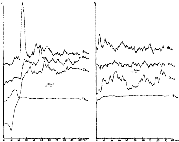
Рис. 6. Изменение интенсивности рентгено-спектральных линий отдельных элементов в стали ШХ-15 после обжаривания. Справа – на краю образца без обжаривания (для оценки «краевого эффекта»)
