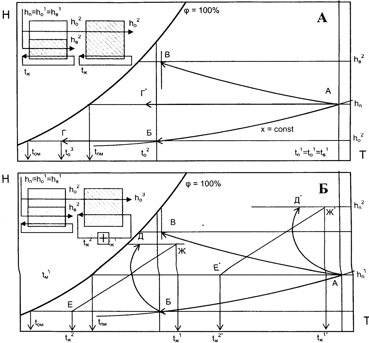
Рис. 5. Изображение процесса в комбинированном охладителе на Н-Т диаграмме влажного воздуха. А – процессы в охладителе на основе НИО/ПИО; Б – процессы в охладителе на основе НИО/ГРД. Обозначения по рисунку 4.4А, дополнительно: БГ и АГ* – процессы в ПИО; ЕЖ и Е*Ж* – рабочие линии градирен; АД* и БД – линии изменения состояния воздуха в градирнях
