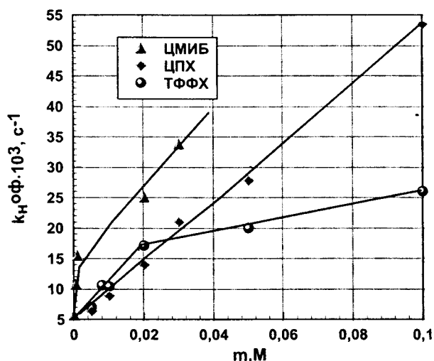
Рис.2. Зависимость наблюдаемых констант скорости реакции (1) в отделенной органической фазе ( k_n^{оф}(c^{-1}) ) от концентрации межфазного катализатора ( m, M )
