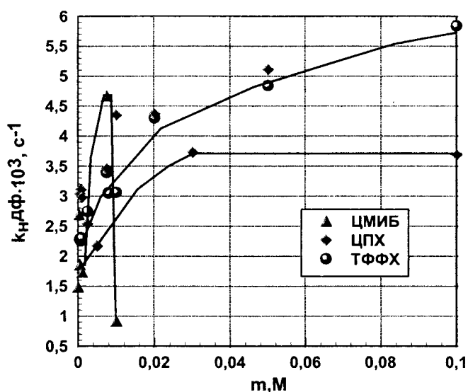
Рис.1. Зависимость наблюдаемых констант скорости реакции (1) в двухфазной системе ( k_n^{дф}(c^{-1}) ) от концентрации межфазного катализатора ( m, M )
