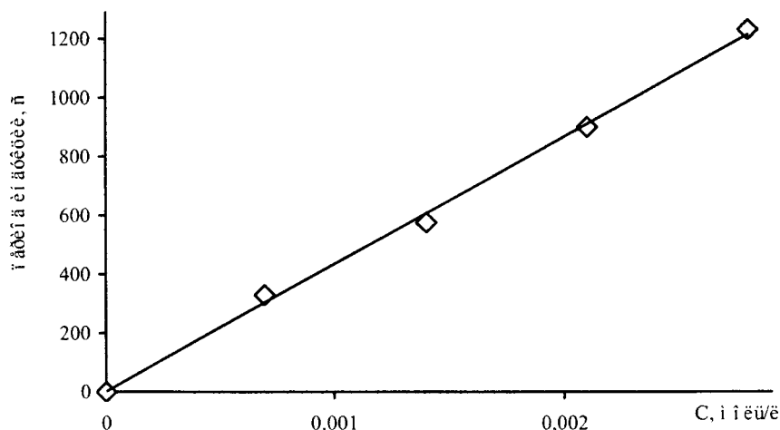
Рис.3. Влияние концентрации антрона в среде ДМСО на период индукции в процессе окисления изопропилбензола при 343 К P_{O_2} = 760 мм рт. ст.: V(\text{ДМСО}) = V(\text{кумола}) = 1 мл, C_0(\text{АИБН}) = 0,026 моль/л
