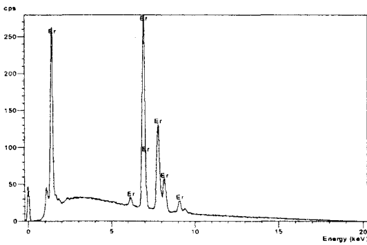
Рис.2а. Состав покрытия эрбия после термической обработки
