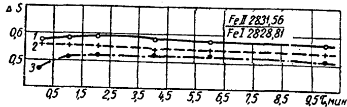
Рис. 5. Изменение \Delta S фиксипар спектральных искровых и дуговых линий отожженных (1), цементованных (2) и азотированных (3) образцов среднелегированных сталей при длительном обжаривании. Искровое возбуждение: U = 12 кВ, C = 0,01 мкФ, L = 0,01 мГн
