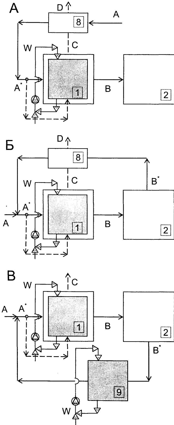
Рис. 2. Примеры использования НИО в составе альтернативных систем (патент Украины № 73696).
