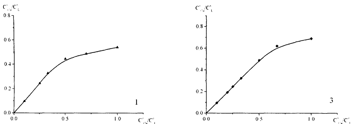
Рис. 1. Криві залежності C_{\text{Cu}}^S/C_L^S від C_{\text{Cu}}^0/C_L^0 для зразків 1 та 3 ( V = 25\text{ cm}^3 , m_{\text{ФМПС}} = 0,3\text{ г} , \tau = 24\text{ год} ) (номер кривої відповідає номеру зразка в табл. 1)
