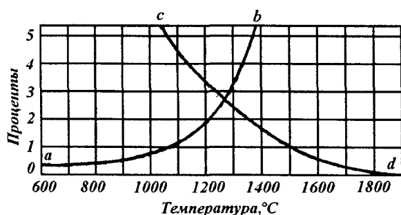
Рис. 11. Влияние температуры на концентрацию углерода в сплавах железо-углерод при их цементации (по Д.К. Чернову) [5]
