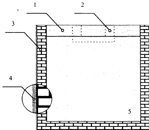
Рис.1 Схематическое изображение ковша. 1 – шлак, 2 – область прохождения тока, 3 – футеровка, 4 – металлический кожух, 5 – расплав
