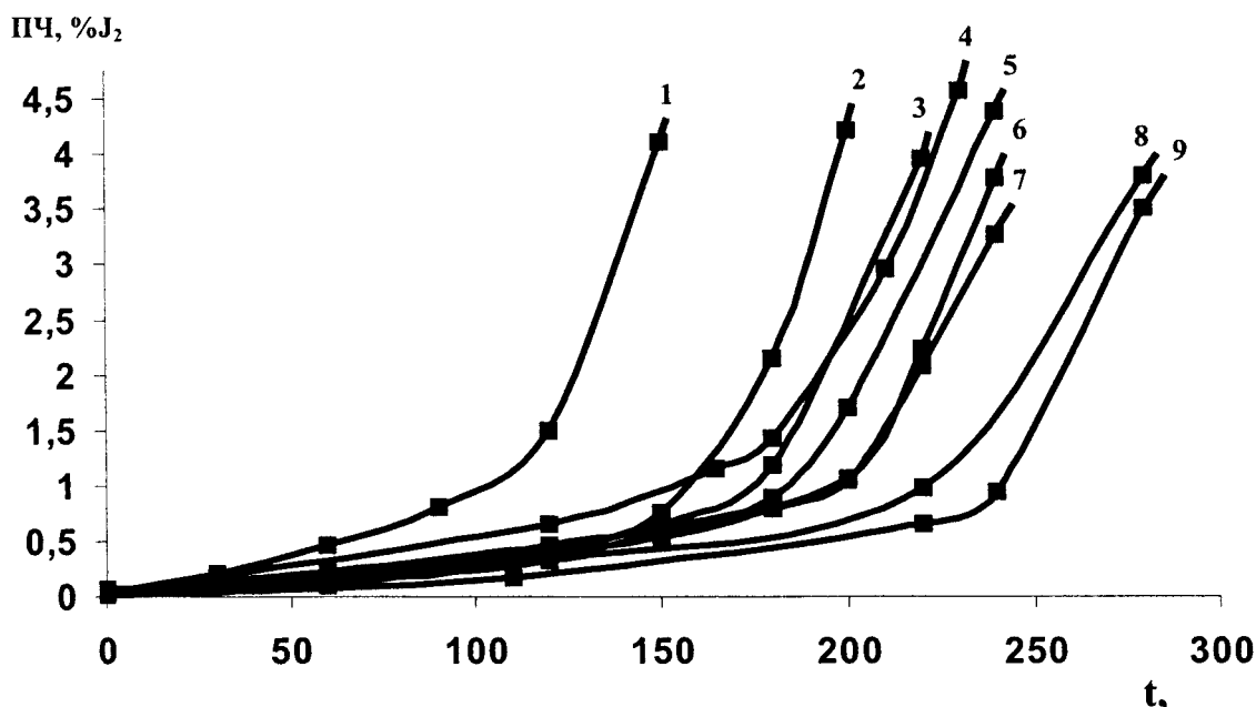
Рис. 2 – Кінетика накоплення пероксидних груп при окисленні сонячного масла (1) при T=393\pm 2K в присутності ПОП (C=10 мас.%) : 2 – чеснок (луковица); 3 – свекла (корнеплод); 4 – хрен (корень); 5 – пастернак (корень); 6 – морква (корнеплод); 7 – перець червоный солоный (мякоть); 8 – салат (листья); 9 – перець жовтий солоный (мякоть).
