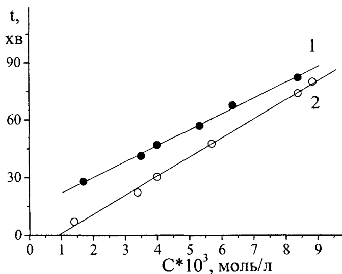
Рис.6. Залежність величини періоду індукції від концентрації аскорбінової кислоти в системі окиснення кумолу киснем при температурі 75^{\circ}\text{C} : 1 – у присутності супероксид-аніона однакових концентрацій; 2 – без супероксид-аніона
