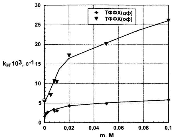
Рис.3. Зависимость наблюдаемых констант скорости реакции (1) в двухфазной системе и отдельной органической фазе от концентрации тетрафенилфосфоний хлорида (m, M)
