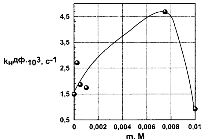
Рис.4. Зависимость наблюдаемых констант скорости реакции (1) в двухфазной системе ( k_{ндф}(c^{-1}) ) от концентрации 1-цетил-3-метилимидазолий бромид ( m, M )
