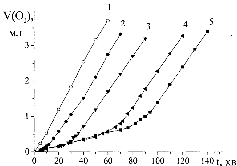
Рис.3. Ініційоване АІБН ( 2,00 \cdot 10^{-2} моль/л) окиснення кумолу в середовищі ацетонітрилу в присутності аскорбінової кислоти при варіюванні її концентрації при постійній температурі 75\text{ }^{\circ}\text{C} : 1 – без аскорбінової кислоти, 2 – 1,40 \cdot 10^{-3} моль/л, 3 – 4,00 \cdot 10^{-3} моль/л, 4 – 5,71 \cdot 10^{-3} моль/л, 5 – 8,40 \cdot 10^{-3} моль/л.
