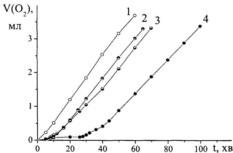
Рис.4. Ініційоване АІБН ( 2,00 \cdot 10^{-2} моль/л) окиснення кумолу киснем в середовищі ацетонітрилу при постійній температурі 75\text{ }^{\circ}\text{C} : 1 – без інгібіторів; 2 – у присутності супероксид-аніона; 3 – у присутності аскорбінової кислоти; 4 – у присутності супероксид-аніона і аскорбінової кислоти
