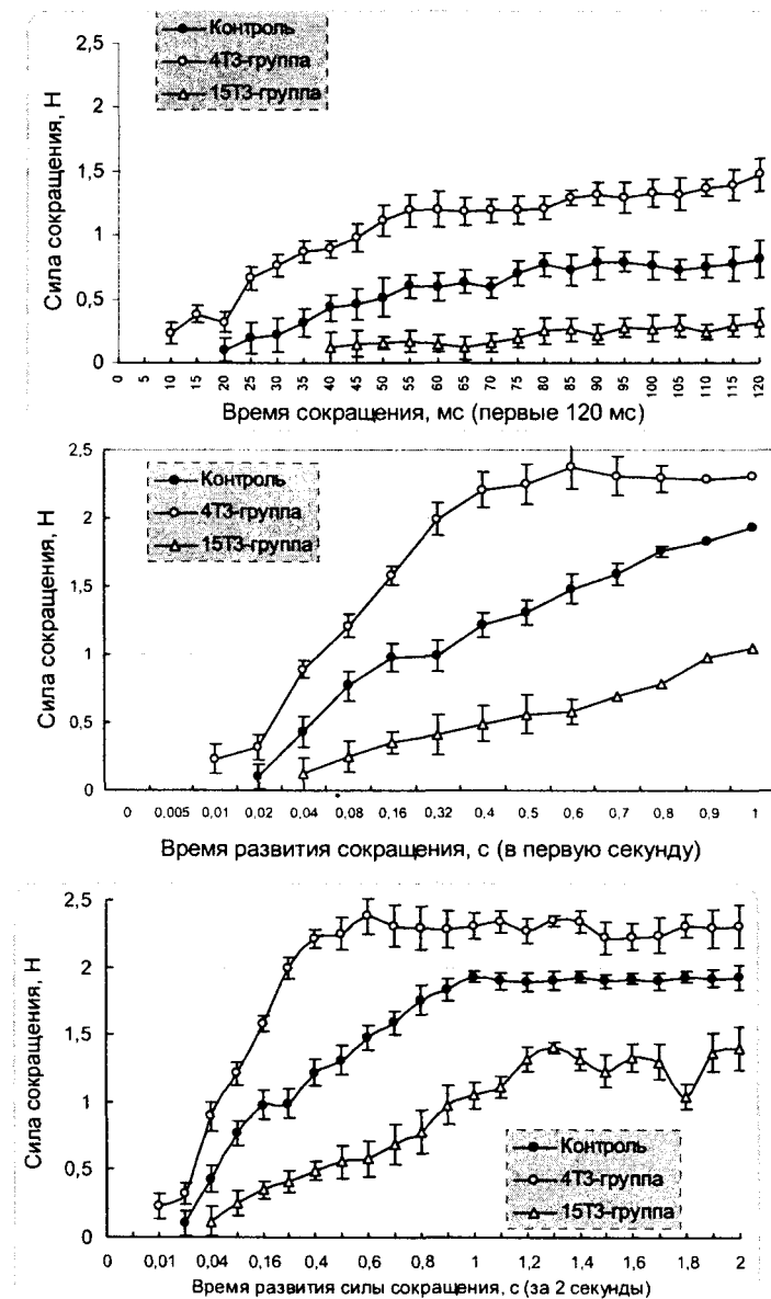
Рис.3. Характер развития сокращения в разные его фазы у крыс контрольной группы и животных, получивших предварительно 4 и 15 инъекций три-йодтиронина
