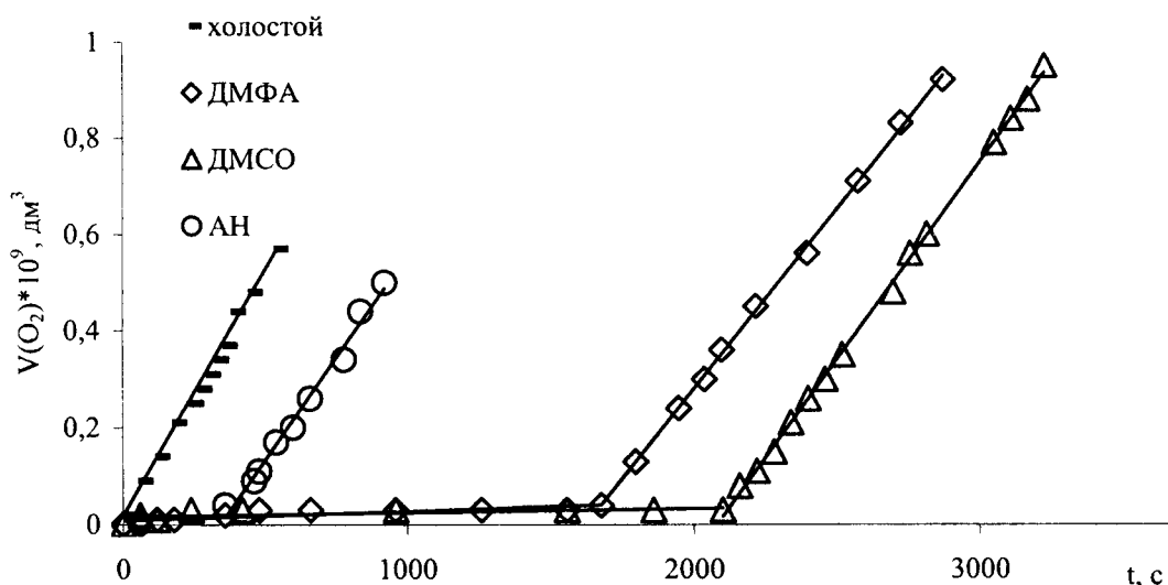
Рис.2. Кинетические кривые поглощения кислорода кумолом в присутствии антрона в ДМСО, ДМФА и АН при 343 К, P O 2 = 760 мм рт.ст.: C 0 (антрона) = 0,003 моль/л, V(ДМСО) = V(ДМФА) = V(АН) = V(кумола) = 1 мл, C 0 (АИБН) = 0,026 моль/л
