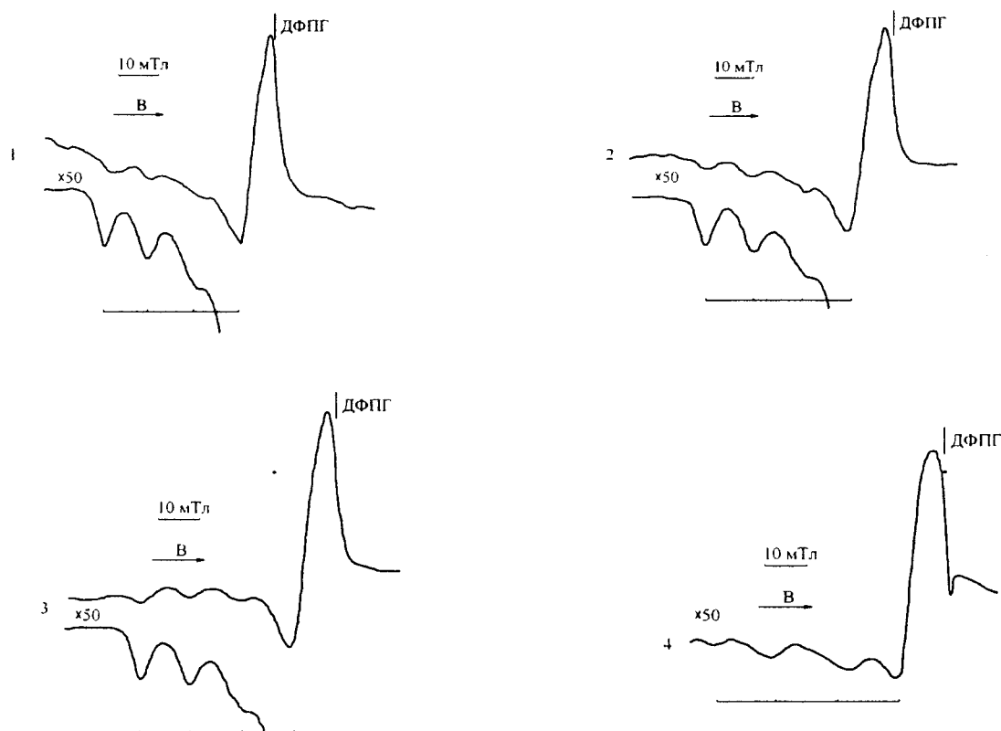
Рис. 4. Спектри ЕПР комплексів міді(II) на поверхні ксерогелю 1 (1 – співвідношення Cu^{2+}/NH_2 = 1:10 , 2 – 1:4, 3 – 1:3, 4 – 1:2).
