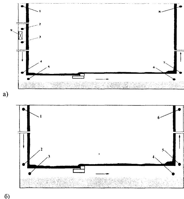
Рис. 1. Схема расположения замерных пунктов и измеряемые параметры вентиляционного воздуха при проведении тепловых съемок на выемочном участке: а – при охлаждении рудничного воздуха; б – без охлаждения рудничного воздуха; 1 – 8 точки замеров тепловлажностных параметров и расхода воздуха; 9 – воздухоохладитель
