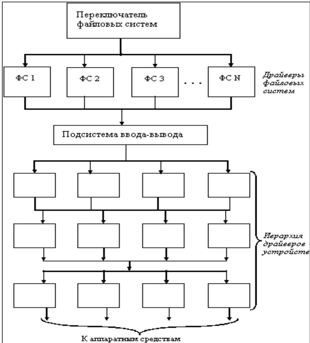
Рис. 11.4. Архитектура современной файловой системы
