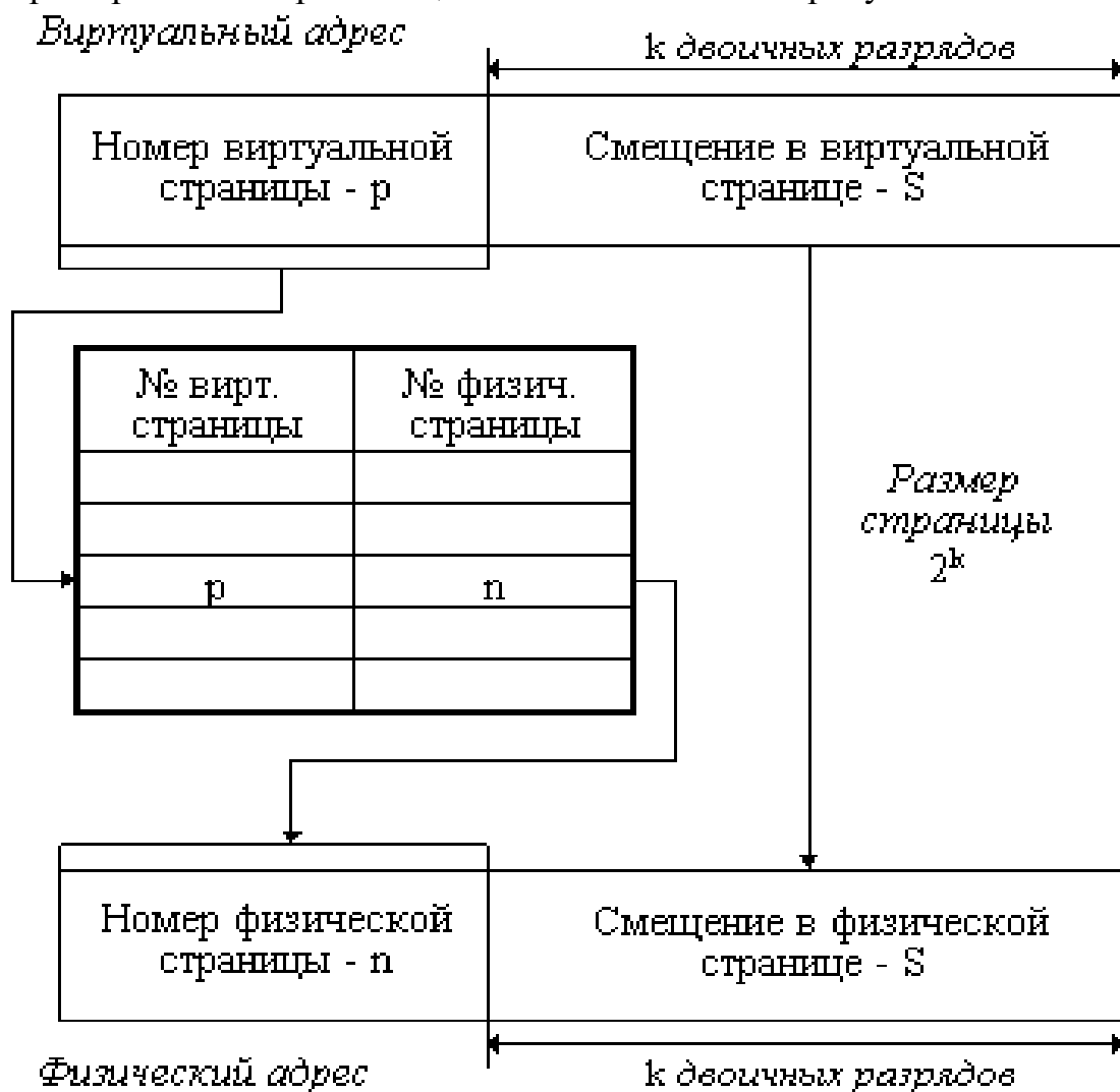
Рис. 7.2. Механизм преобразования виртуального адреса в физический адрес при страничной организации памяти
