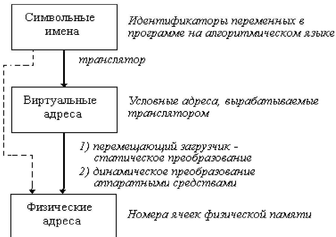
Рис. 6.1. Типы адресов
