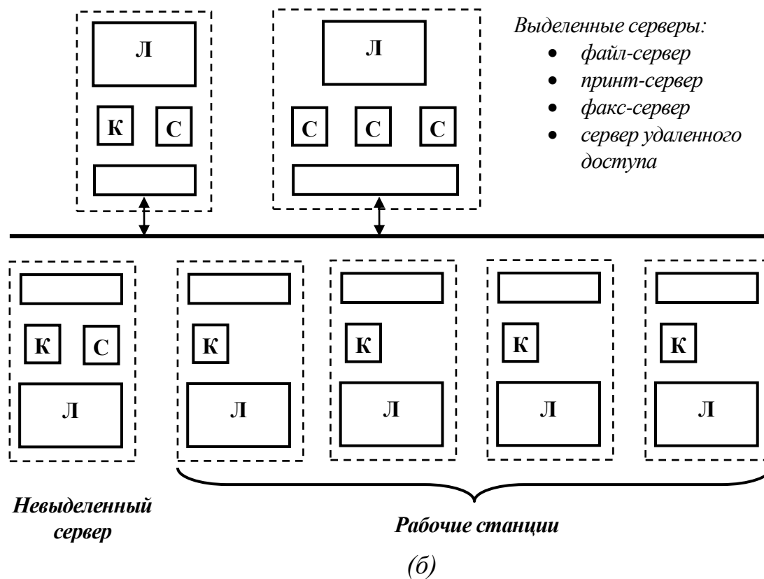
Рис. 2.4. (а) – Одноранговая сеть (б) – Двухранговая сеть
