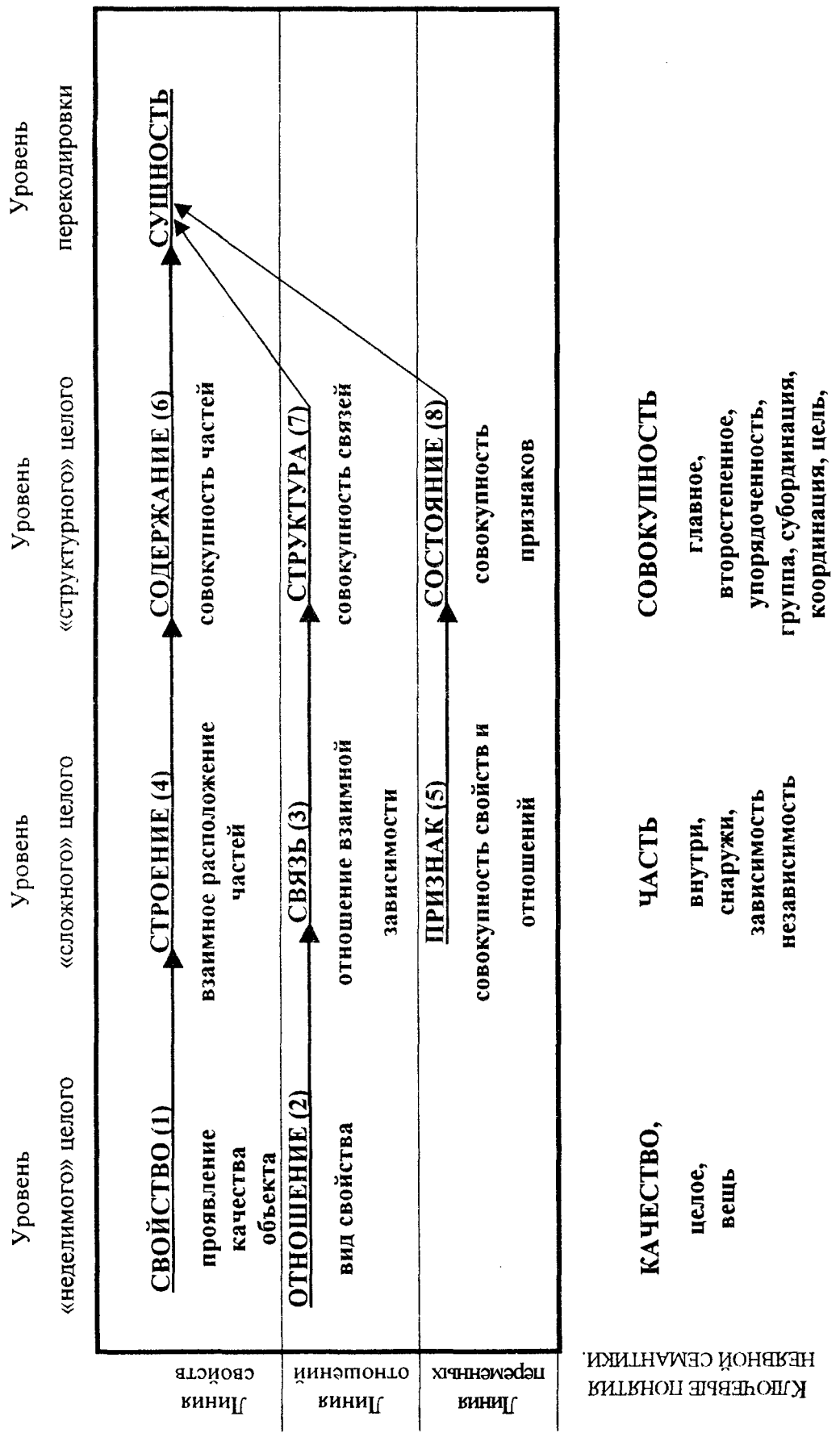
Рис. 1. Структура «сущности»
