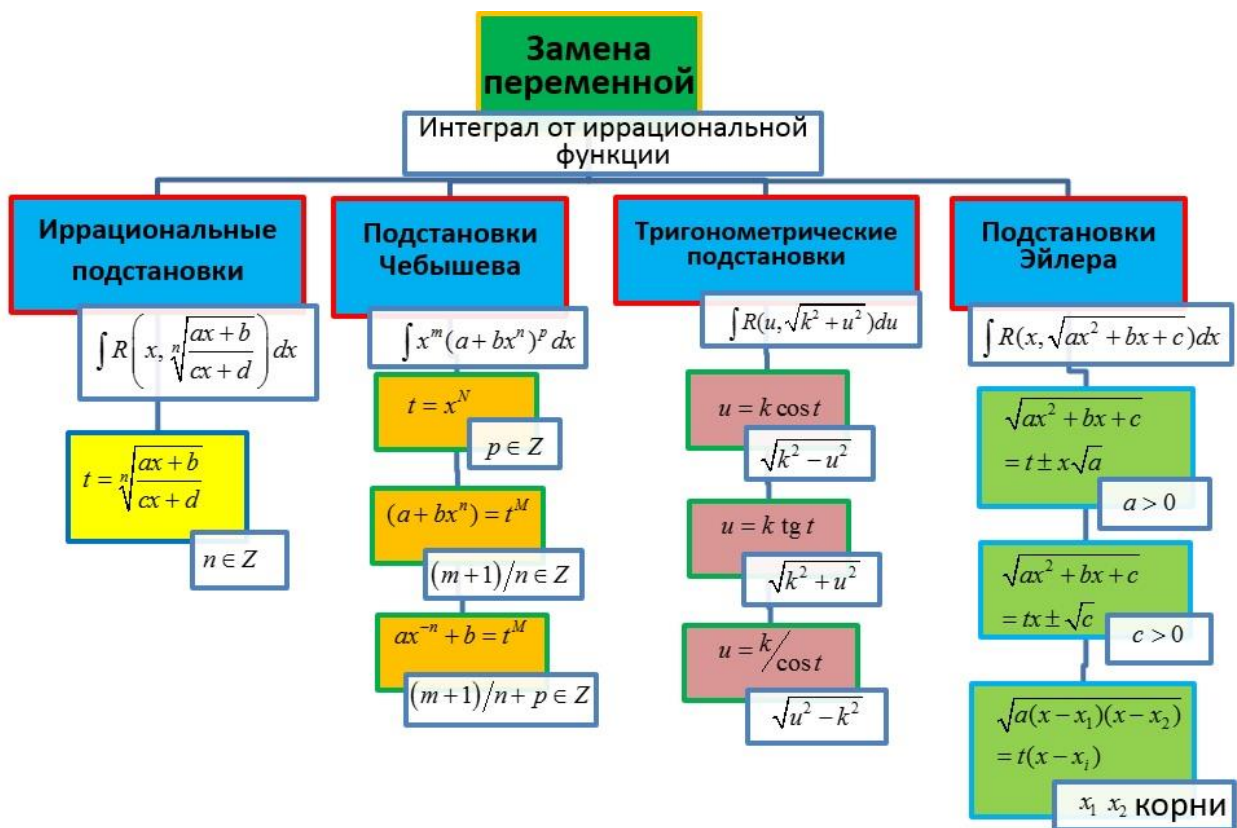
Рисунок 4.4 – Логический граф классификации приемов интегрирования иррациональной функции с использованием метода замены переменной
