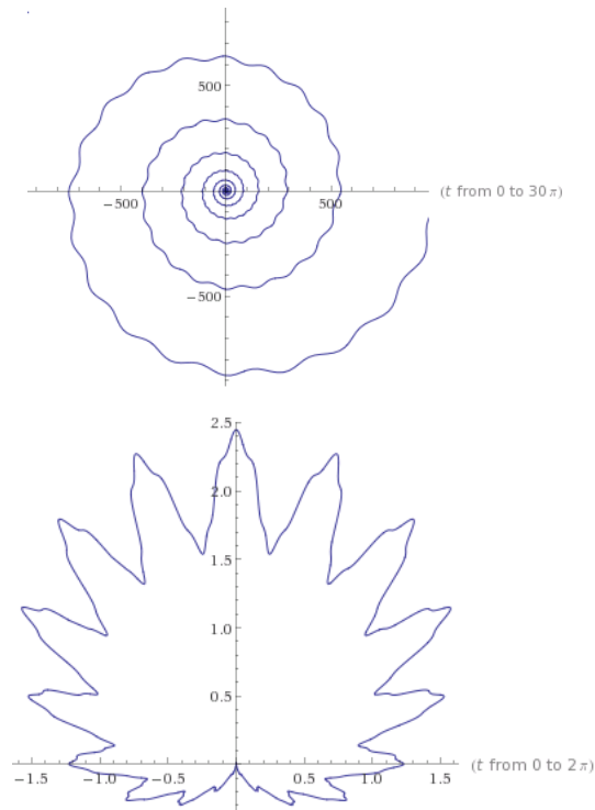
Рисунок 1 – Графики функций
