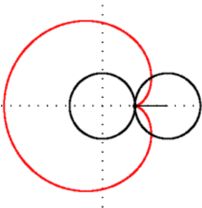
Рисунок 4.2 – Кардиоида кардиоиды (Рисунок 4.2).
