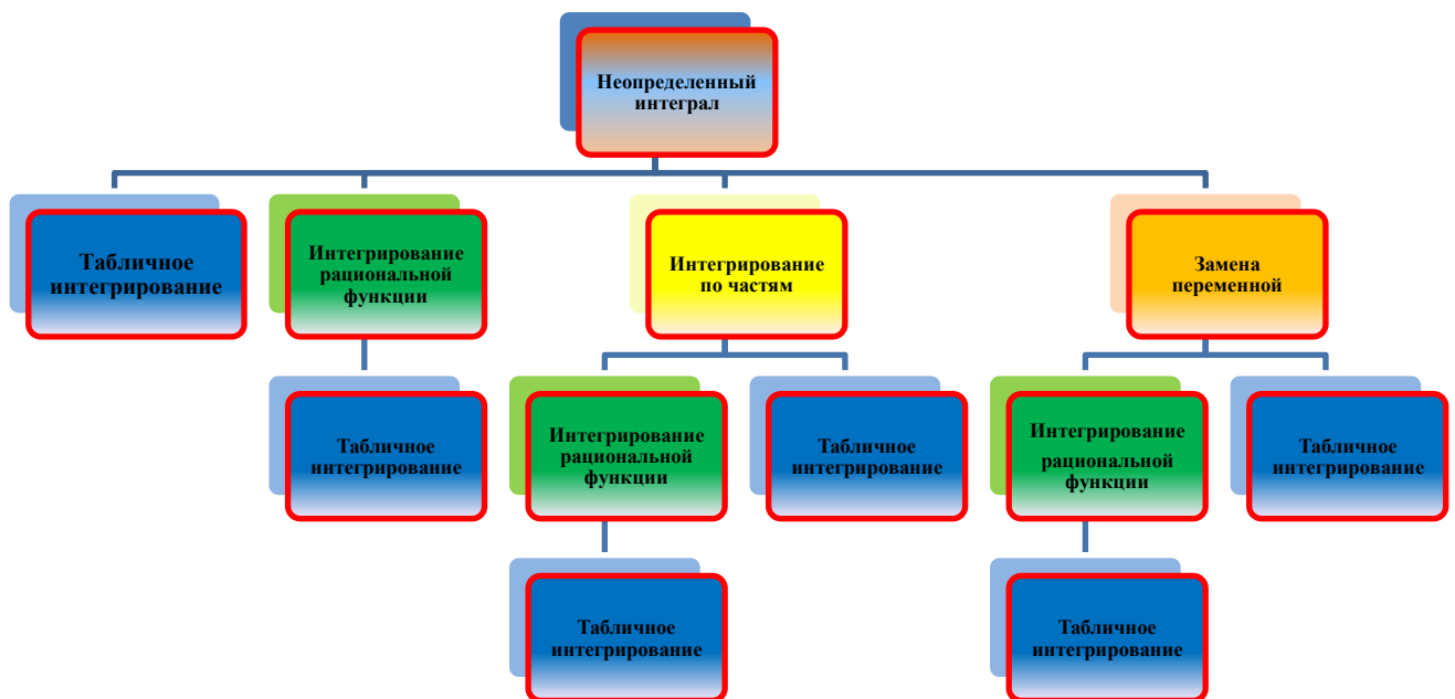
Рисунок 3.2 – Логический блок классификации подходов к вычислению неопределенного интеграла
