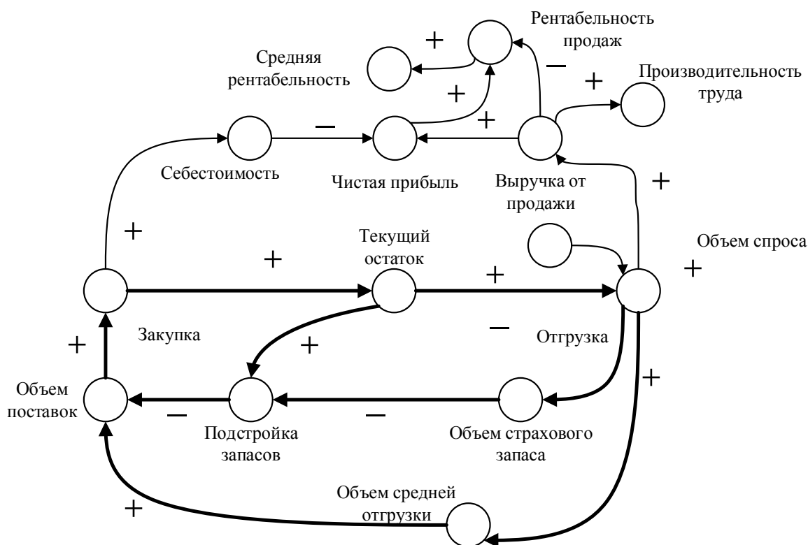
Рис. 3. Диаграмма причинно-следственных связей системно-динамической модели оценки эффективности логистической деятельности предприятия оптово-розничной торговли
