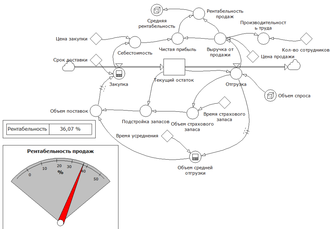
Рис. 4. Системно-динамическая модель оценки эффективности логистической деятельности предприятия оптово-розничной торговли
