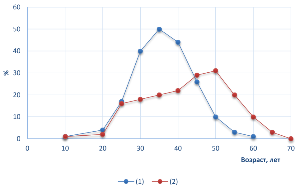
Рис. 3 Распределение выделенных кластеров горнорабочих по возрасту
