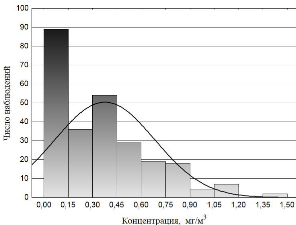
Рисунок 3.1. – Гистограмма плотности вероятности эмпирической функции распределения концентрации диоксида азота на посту № 5 при загрязнении атмосферного воздуха в г. Донецк в 2003 году
